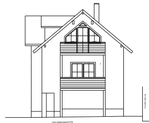
Seitenansicht rechts M:1:100
