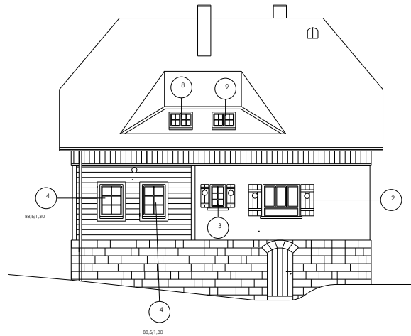
Südansicht
