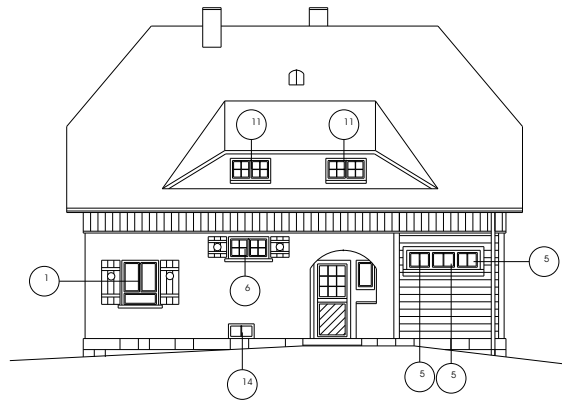
Südansicht
