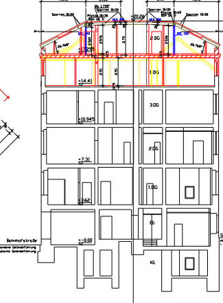
Schnitt A-A M 1:100
