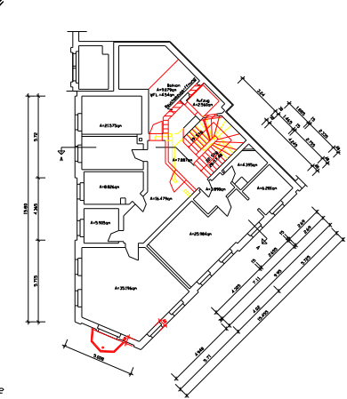
Grundriss 3.OG M 1:100
