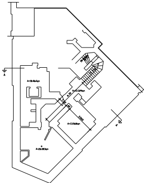
Grundriss 1.OG M 1:100
