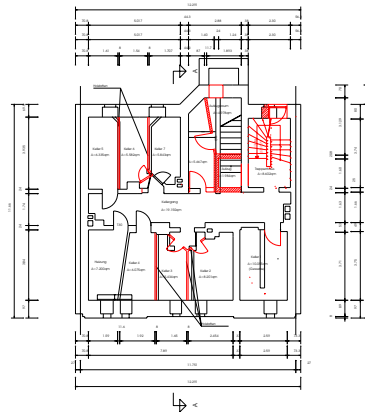
Kellergeschoß M:1:100
