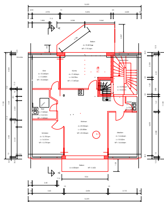
Grundriß 2. Dachgeschoß M:1:100
